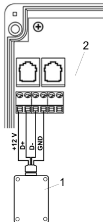
Podłączenie modułu do regulatora głównego SCONTROL MK1 : 1 - moduł radiowy, 2 - regulator główny.
