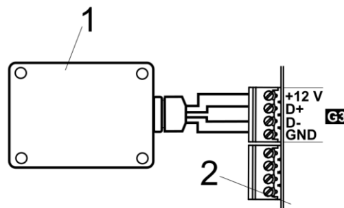
Podłączenie modułu do SCONTROL 910 : 1 - moduł radiowy, 2 - regulator główny.
