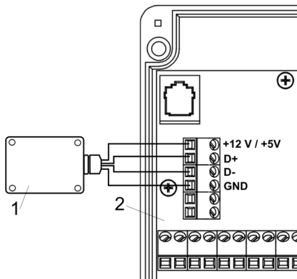
Podłączenie modułu do regulatora głównego RCONTROL 890, 891, 892, SCONTROL 892 : 1 - moduł radiowy, 2 - regulator główny.
